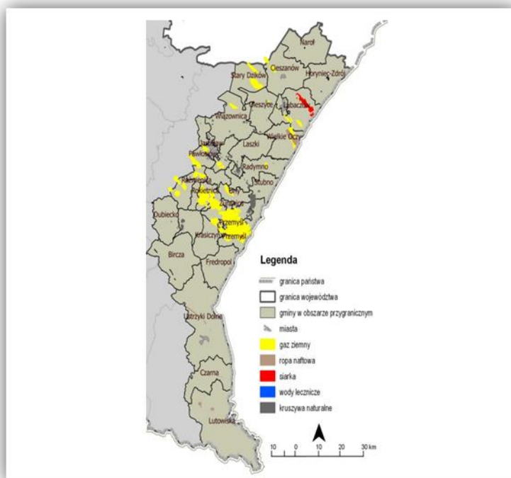
Rycina 1. Rozmieszczenie złóż kopalin na obszarze przygranicznym (wg stanu w 2013 r.)
